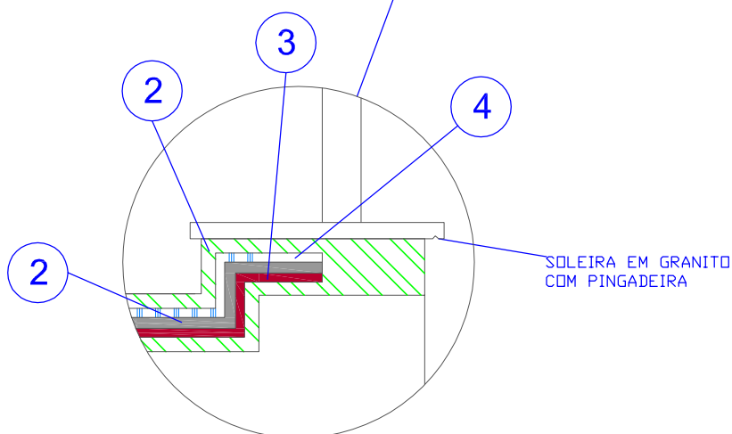
DETALHE SOLEIRA VARANDA
