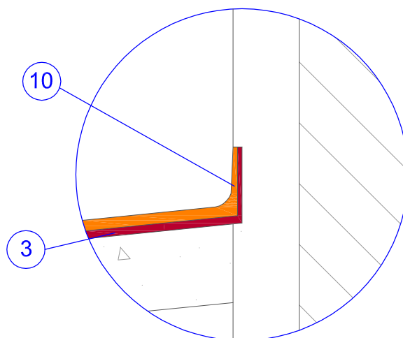
DETALHE ENGASTE NA PAREDE
